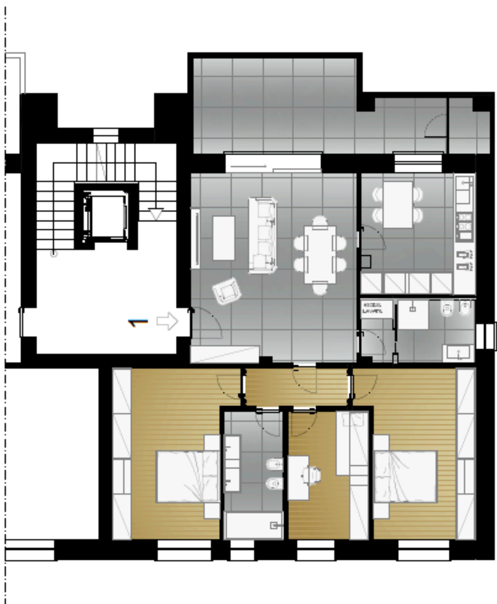
PIANTA PIANO PRIMO - APPARTAMENTO 1
